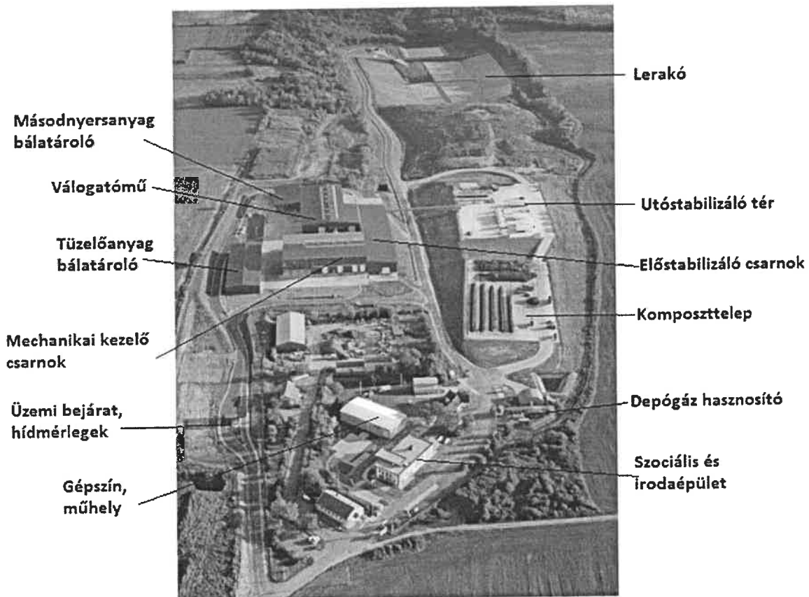
1. ábra: Kökényi Regionális Hulladékkezelő Központ
