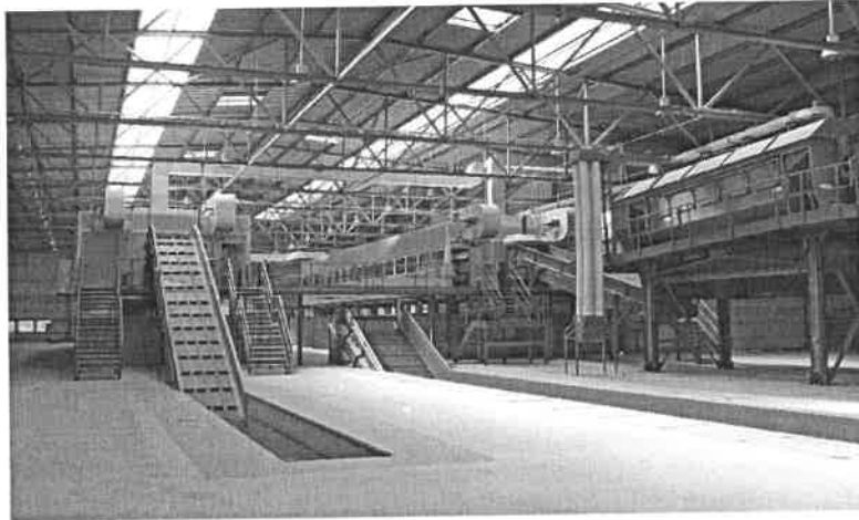
4. ábra: Kökényi válogatómű
